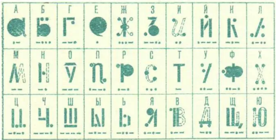
Рис. 1. Азбука Морзе
